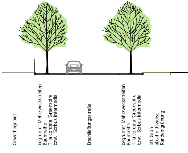
Schnitt 2 M 1:250
